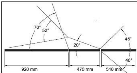
Negativlage bei Option 3-teiliges Kopfteil max. -30°
